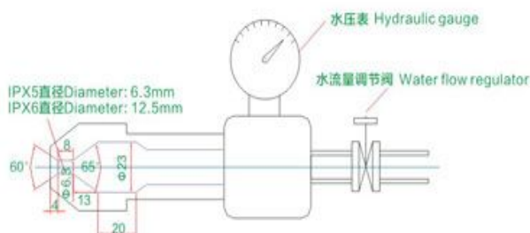
IPX5冲水Flushing IPX6冲水Flushing
